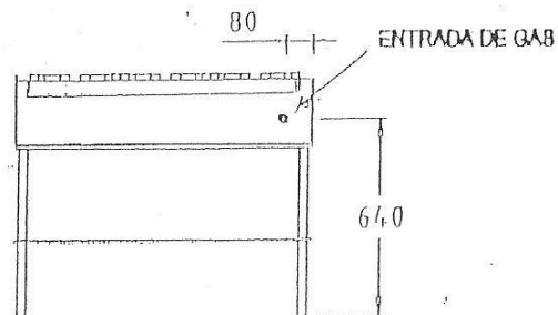
VISTA POSTERIOR MECHERO # 9 MECHERO # 11 MECHERO # 14.5 CONEXION 1" GAS PERILLAS DE BAQUELITA
